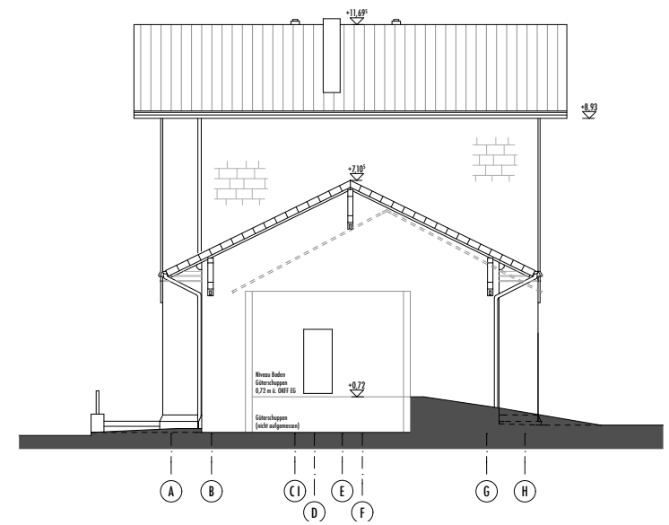
West- Ansicht - M 1|200
