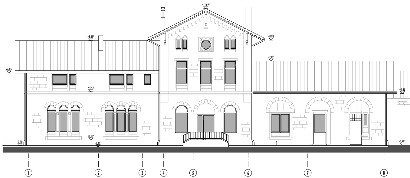
Nord- Ansicht - M 1|200
