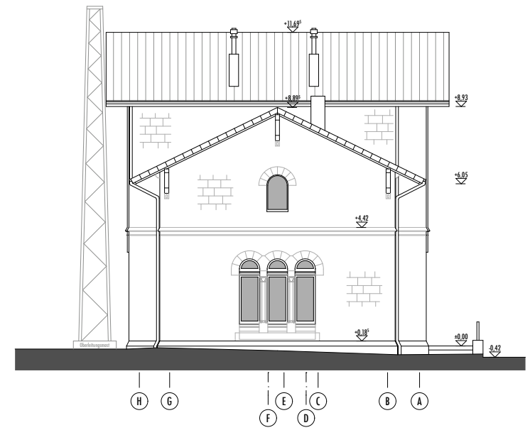
Ost- Ansicht - M 1|200
